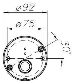
PLANTILLA DE INSTALACIÓN INSTALLATION TEMPLATE
